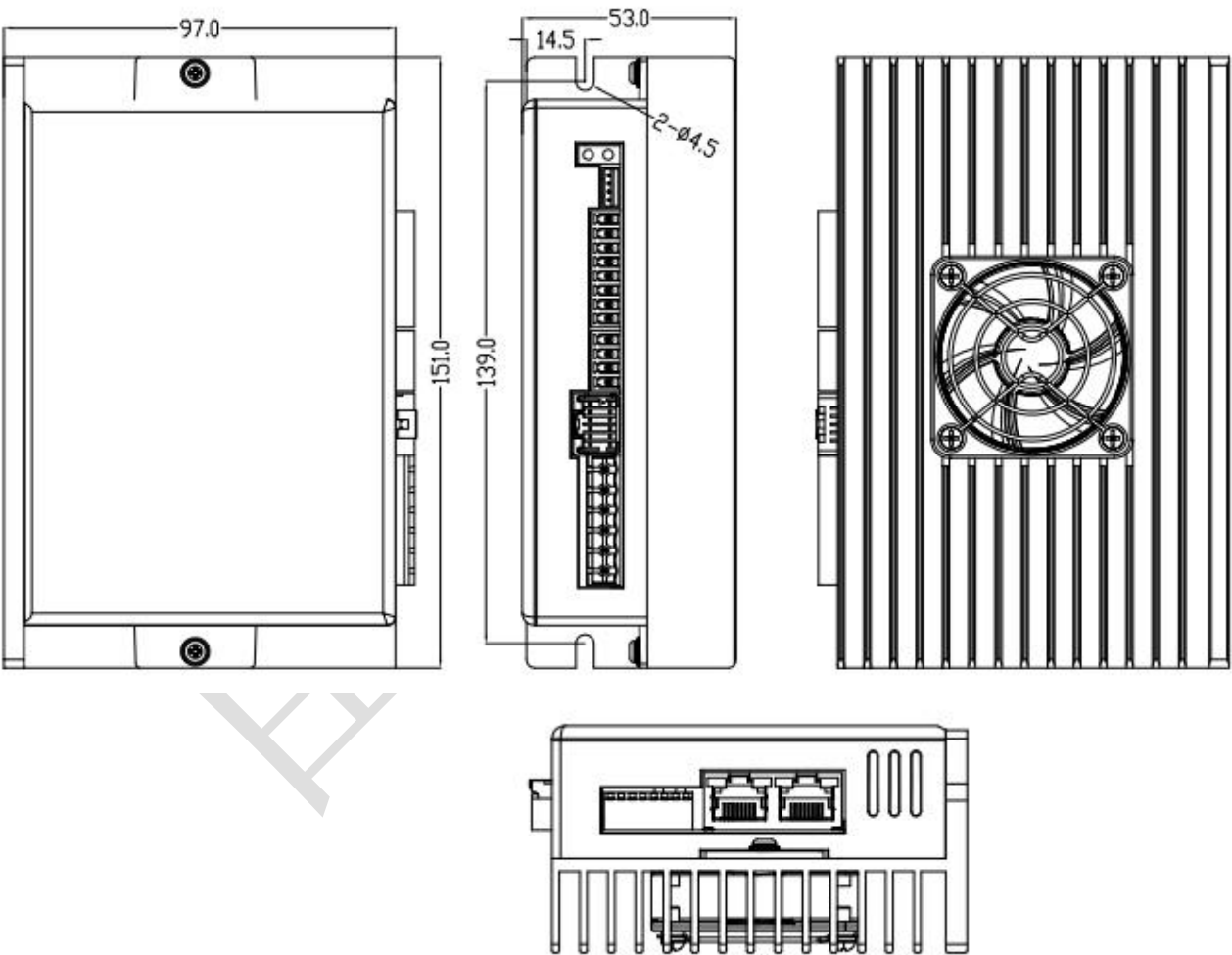
图 2-1 DM2B-RS882AC 驱动器机械尺寸
